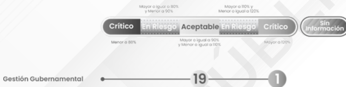
Gráfico 2. Comportamiento de los indicadores de los Pp 2023
